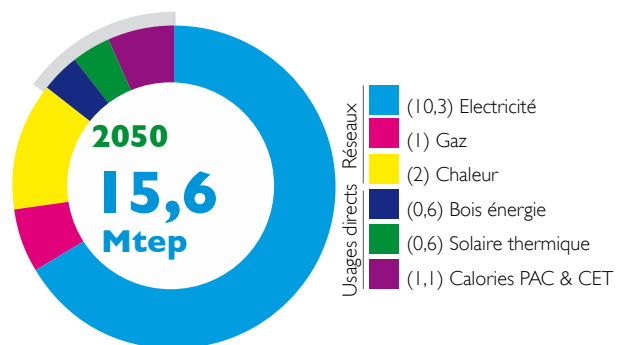
BILAN ÉNERGÉTIQUE DU TERTIAIRE EN 2050, PAR VECTEUR
